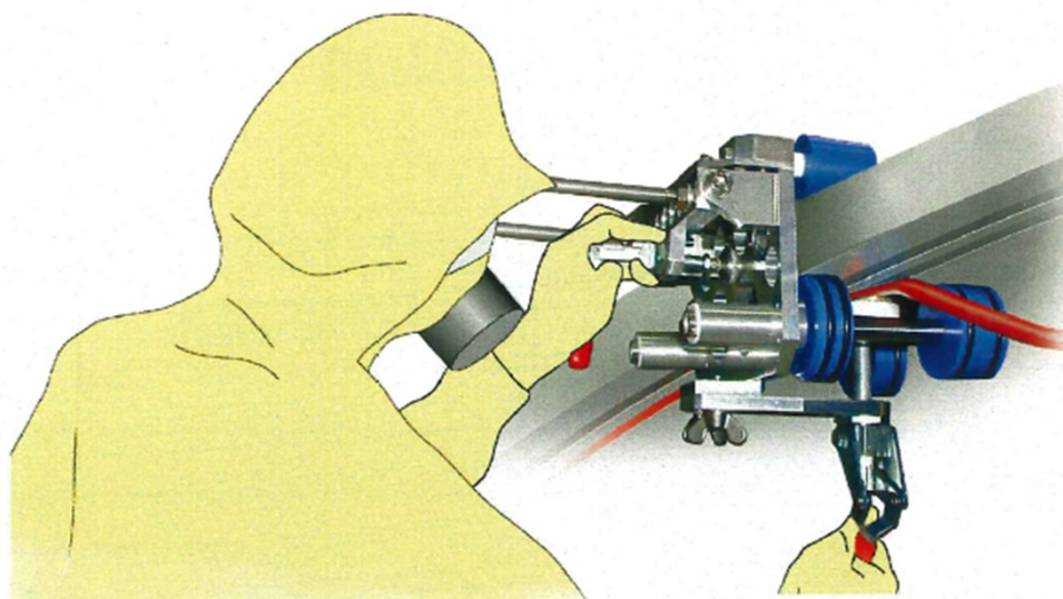
RVシールプレートOリング取付け治具
