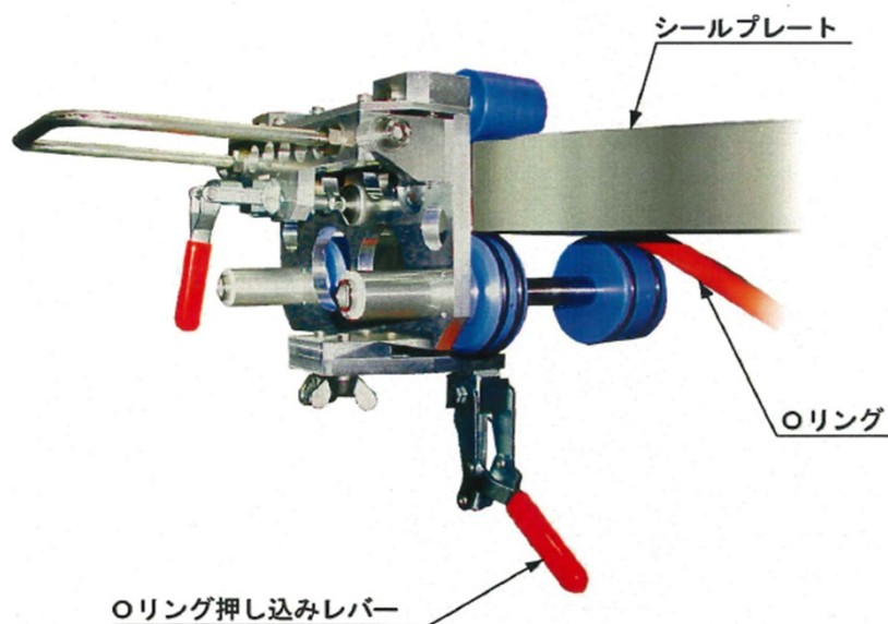
RVシールプレートOリング取付け治具
