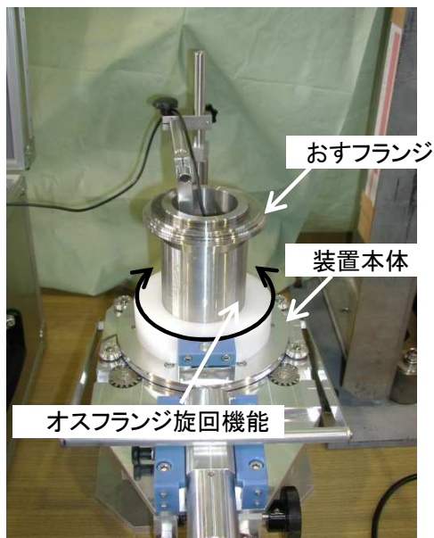
おすフランジコノシール部点検状況 おすフランジを回転させてTCコノシール部を点検します。
