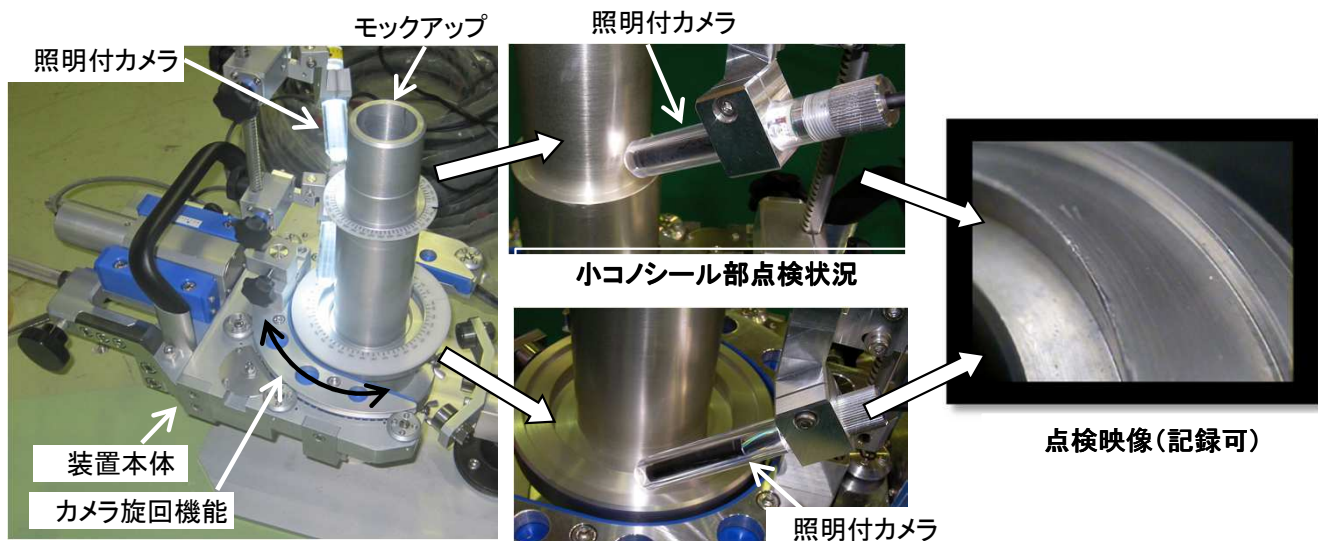
TCコノシール部点検状況 カメラを回転させてTCコノシール部を点検します。 大コノシール部点検状況
