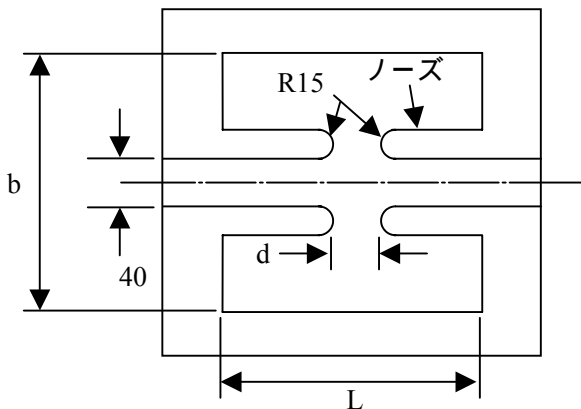
図1：空胴構造
