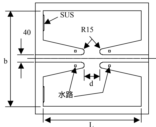
図2：空胴構造(検討後)
