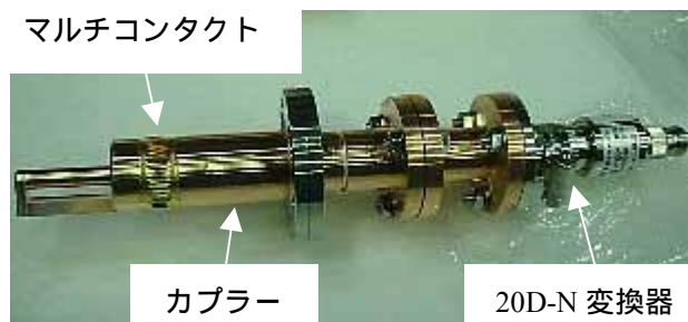
図7：カプラー
