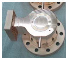
図4：モードコンバータろう付け品
