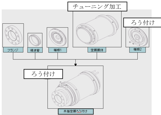
図2：共振空洞製作フロー図
