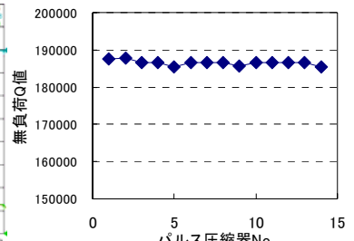
図8：14号機までの無負荷Q値
