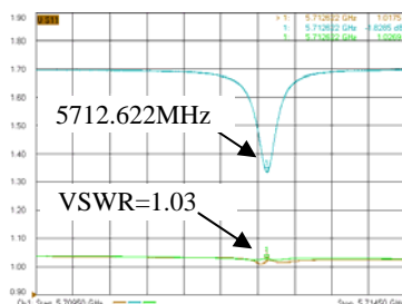
図7：パルス圧縮器RF特性
