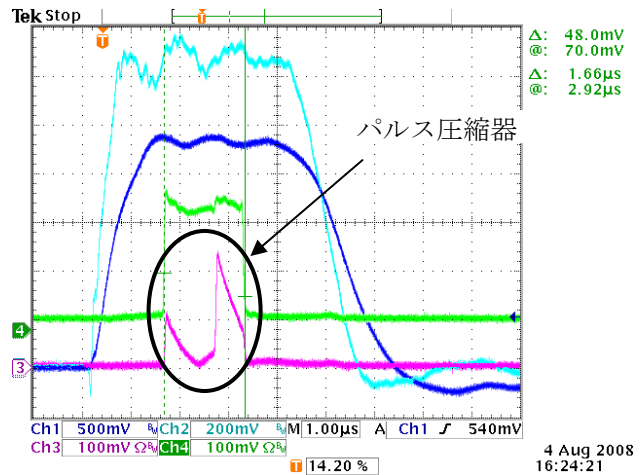
図12：パルス圧縮器高電圧試験結果
