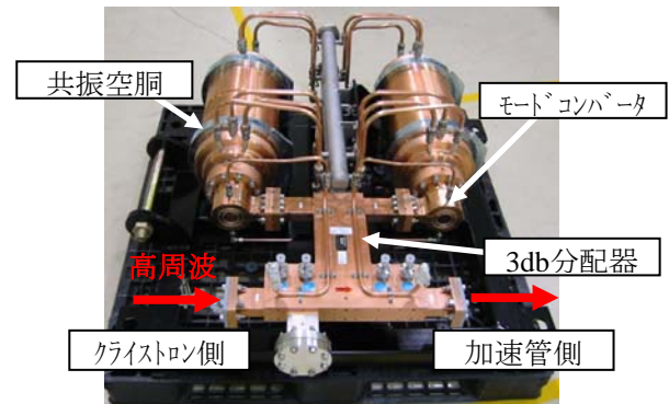
図1: パルス圧縮器
