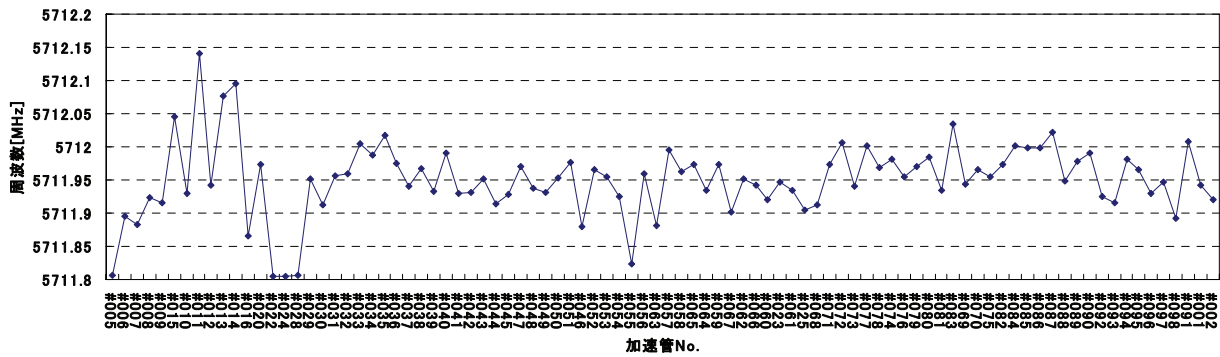
図4：加速管の中心周波数一覧
