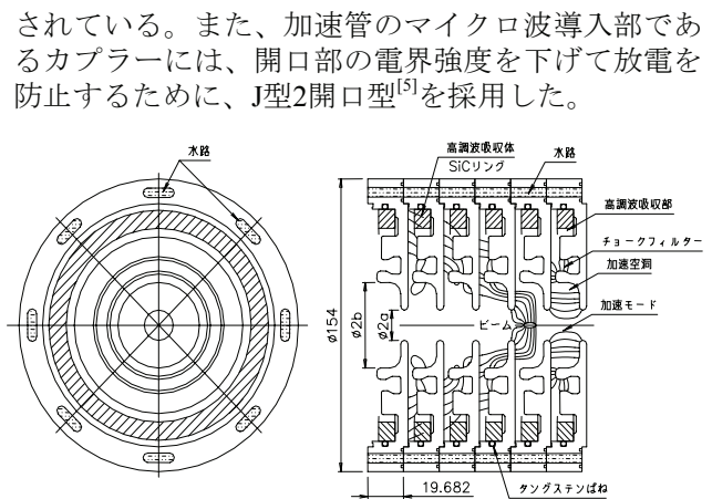
図1: チョーク型加速構造
