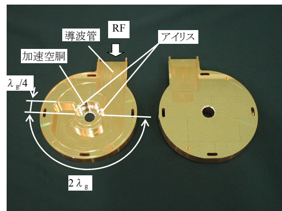
図2: J型2開口型カップラー
