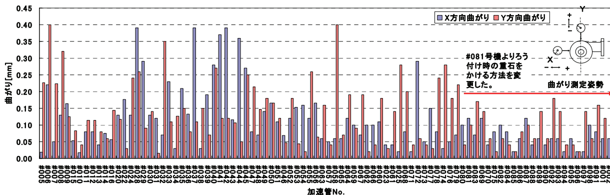
図7：加速管の曲がり一覧
