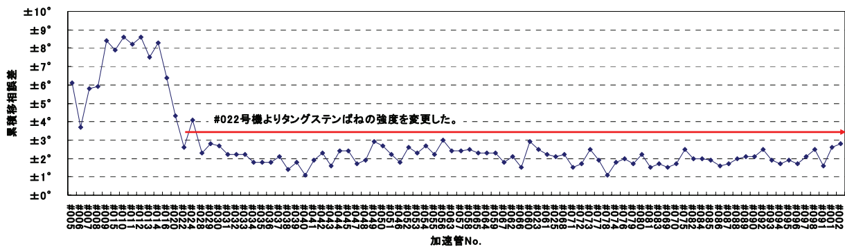
図5：加速管の累積移相誤差一覧
