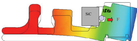
図3：加速管セルの変形状況
