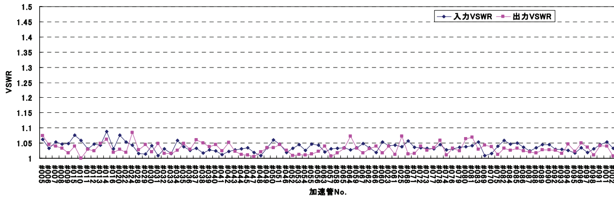
図6：加速管のVSWR一覧
